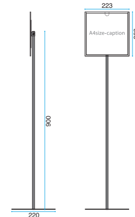
minimum stand | A4 type | スタンド型 A4 タイプ
