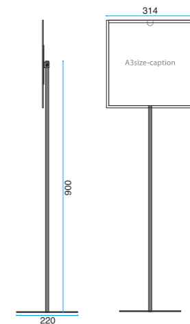
minimum stand | A3 type | スタンド型 A3 タイプ
