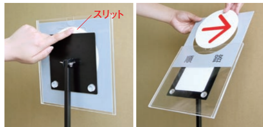
いたずら防止にも一役。裏側のスリットで簡単に矢印の方向が換えられます。
